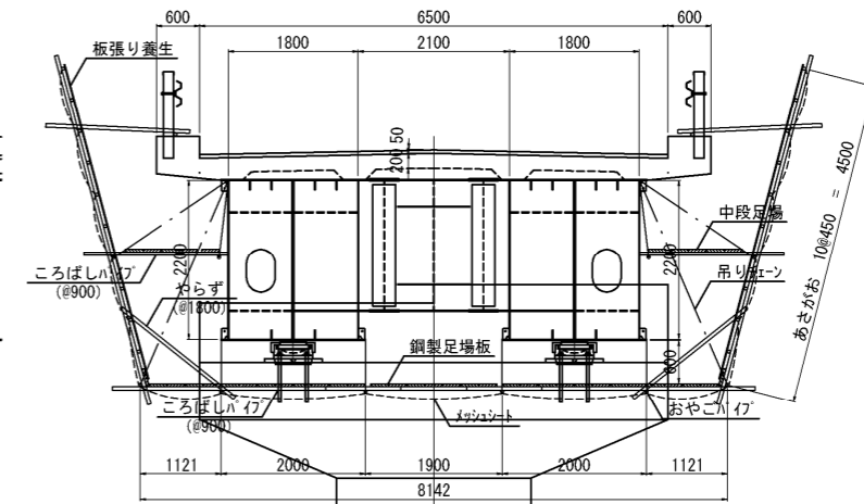
中央径間断面図
