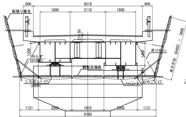
側径間断面図
