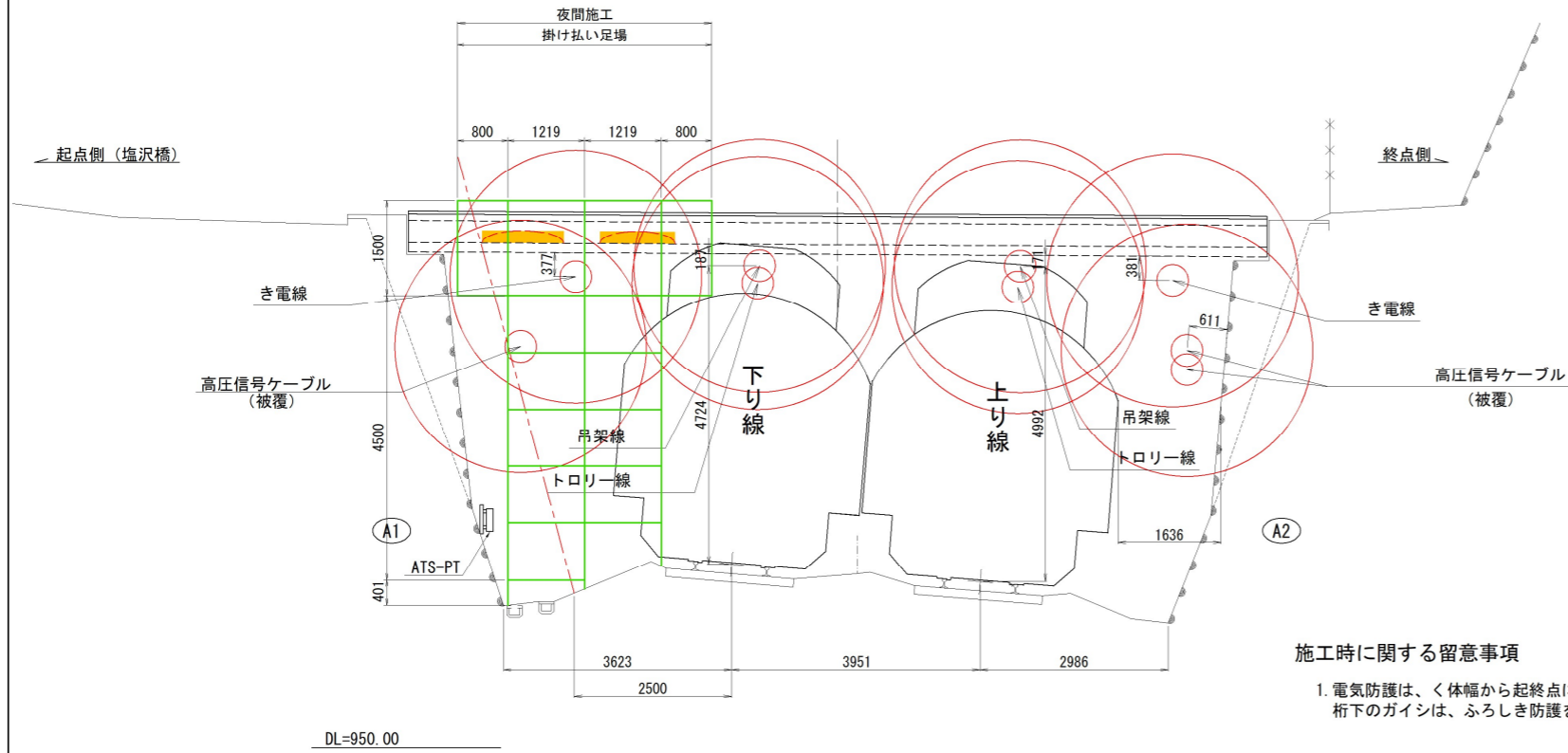
側面図
